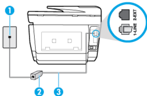
Afbeelding 5-2 Achteraanzicht van de printer
